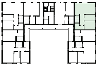
Yfirlitsmynd 1. hæð
