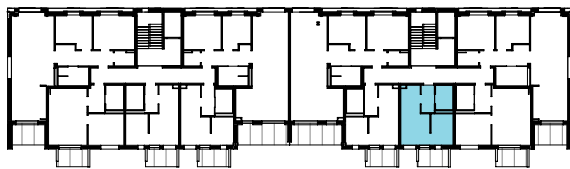
Yfirlitsmynd 5. hæð
